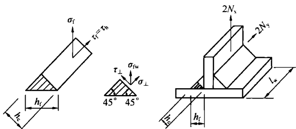
图 11 角焊缝的计算
