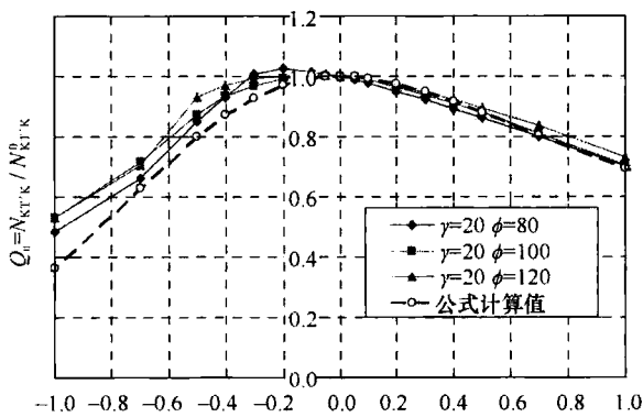
(a) Q_n - n_{TK} 曲线 I
