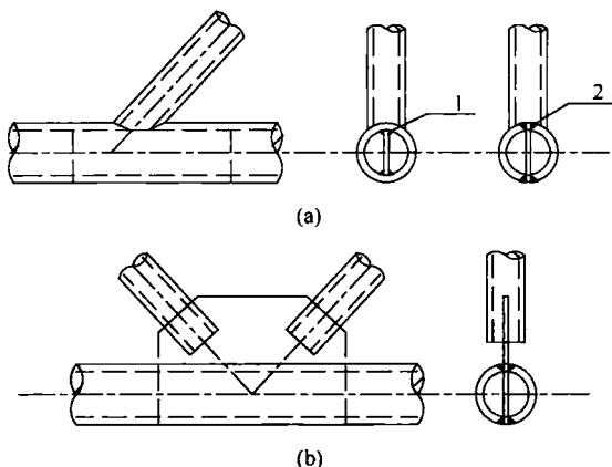
图 34 主管内纵向加劲的节点
