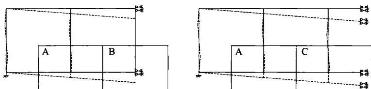
图 53 空腹格构梁的变形模式
