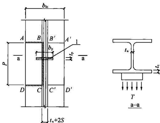
图 18 柱翼缘受力示意
