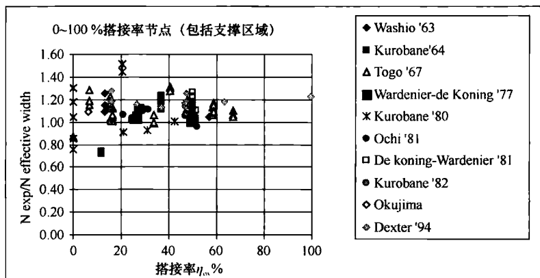
图 30 搭接率对节点承载力的影响
