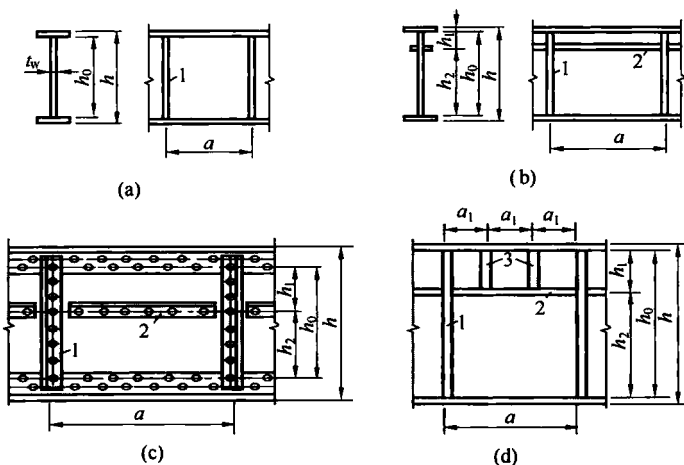
图 6.3.2 加劲肋布置
