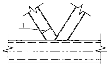
图 33 隐蔽部分施焊时搭接支管断开示意
