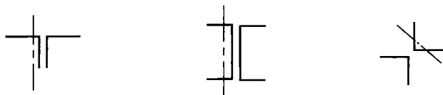
(c) 十字形双角钢截面
