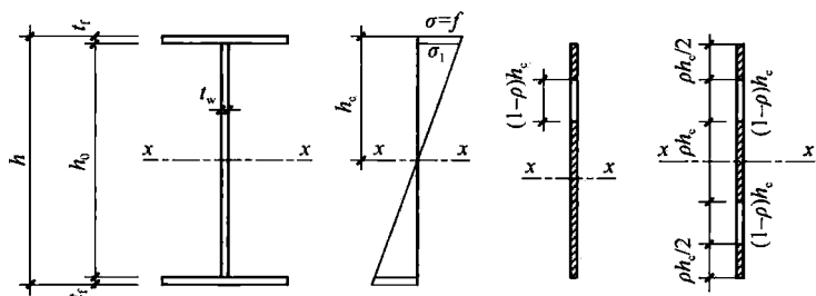
图5 梁截面模量折减系数简化计算简图
