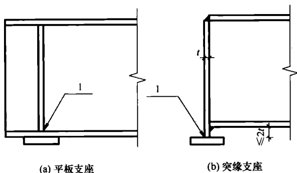
图 12.6.1 梁的支座
