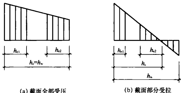
图 8.4.2 有效宽度的分布
