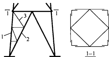
图 7.5.3 塔架下端示意图 1—主杆；2—主斜杆；3—辅助杆
