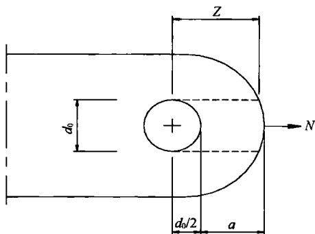
图 11.6.3 销轴连接耳板受剪面示意图
