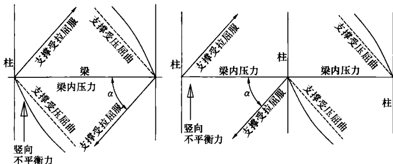
图 49 交叉支撑节点不平衡力示意
