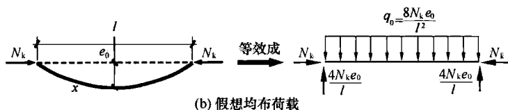
(b) 假想均布荷载
