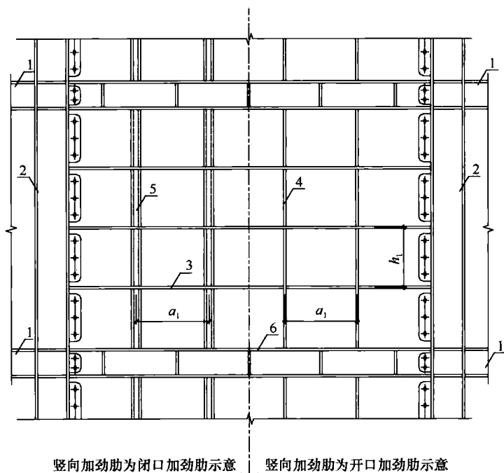
图 10 加劲钢板剪力墙示意
