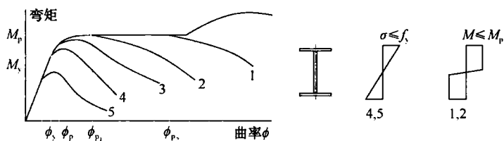
图 1 截面的分类及其转动能力
