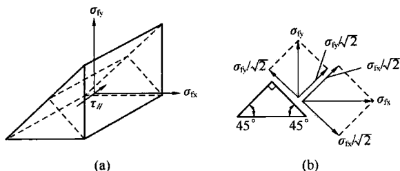
图 12 角焊缝 \sigma_{fx} 、 \sigma_{fy} 、 \tau_{fz} 共同作用
