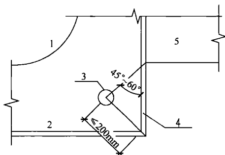
图 45 矩形钢管混凝土柱隔板开孔
