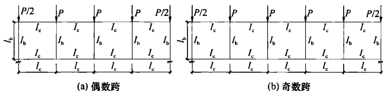
图 52 多跨空腹桁架
