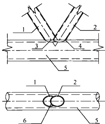
图 31 搭接连接的隐蔽部位
