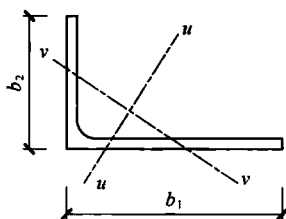
图 7.2.2-2 不等边角钢
