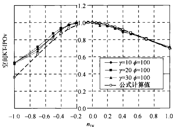
(b) Q_n - n_{TK} 曲线 II
