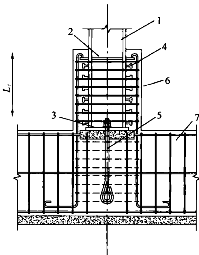
图 12.7.7 外包式柱脚
