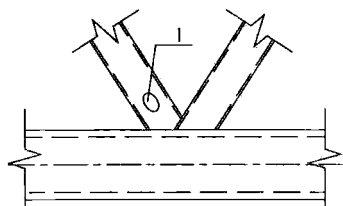
图 32 焊接手孔示意
