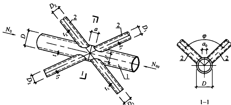
图 13.3.3-2 空间 KK 形节点
