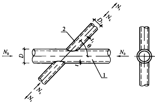
图 13.3.2-1 X 形节点
