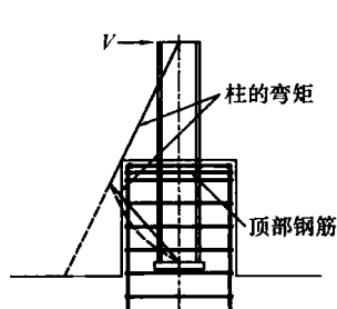
图 20 外包式柱脚的弯矩
