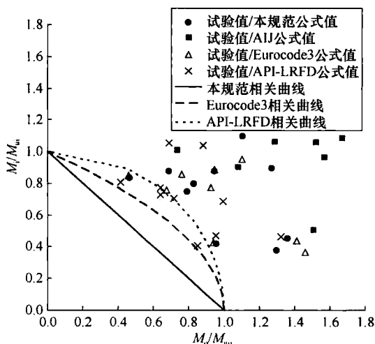
图 42 M_i - M_o 相关方程与试验数据的比较
