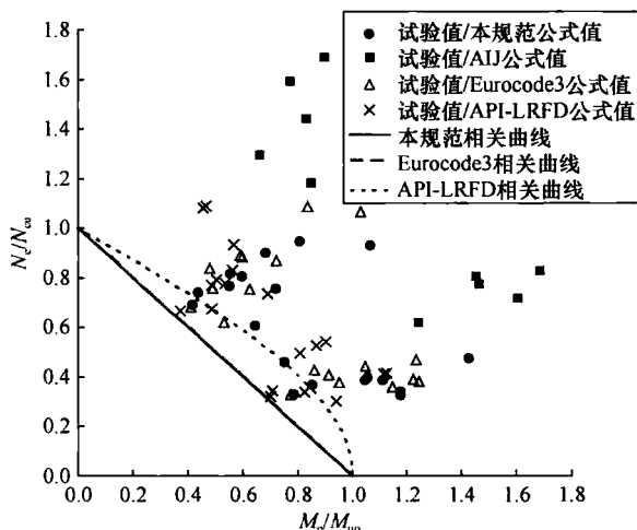
图 40 N_c - M_o 相关方程与试验数据的比较
