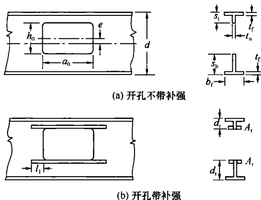
图 6 腹板开孔梁计算几何图形
