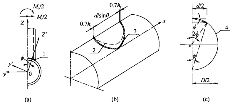
图 43 焊缝截面的简化
