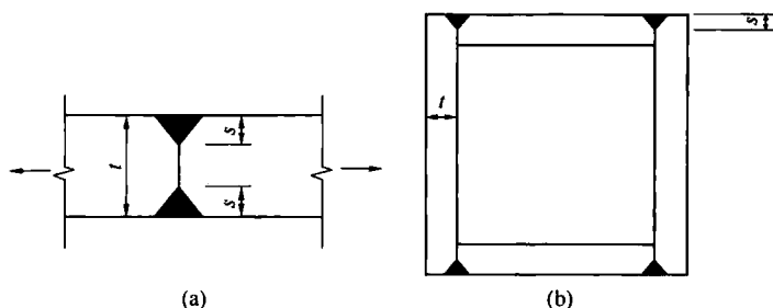
图 14 部分焊透的对接焊
