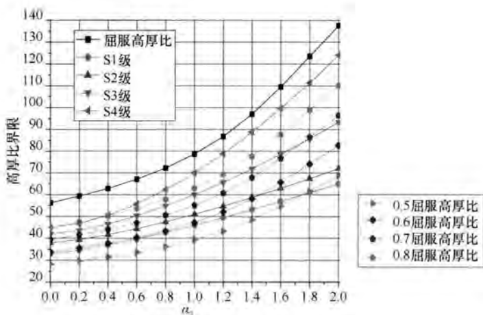
图2 腹板分级的界限高厚比的对比
