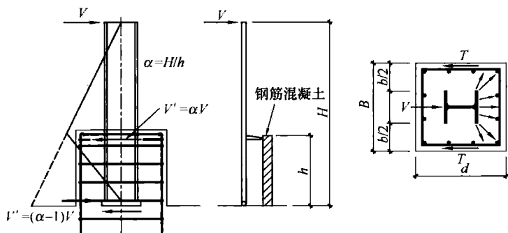
图 23 外包式柱脚的计算概念图
