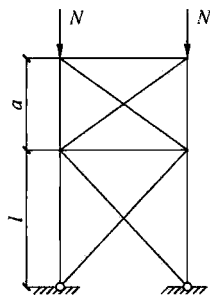
图 8 有支撑的二段柱
