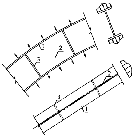
图7 弧曲杆受力示意 (上翼缘受压下翼缘受拉)
