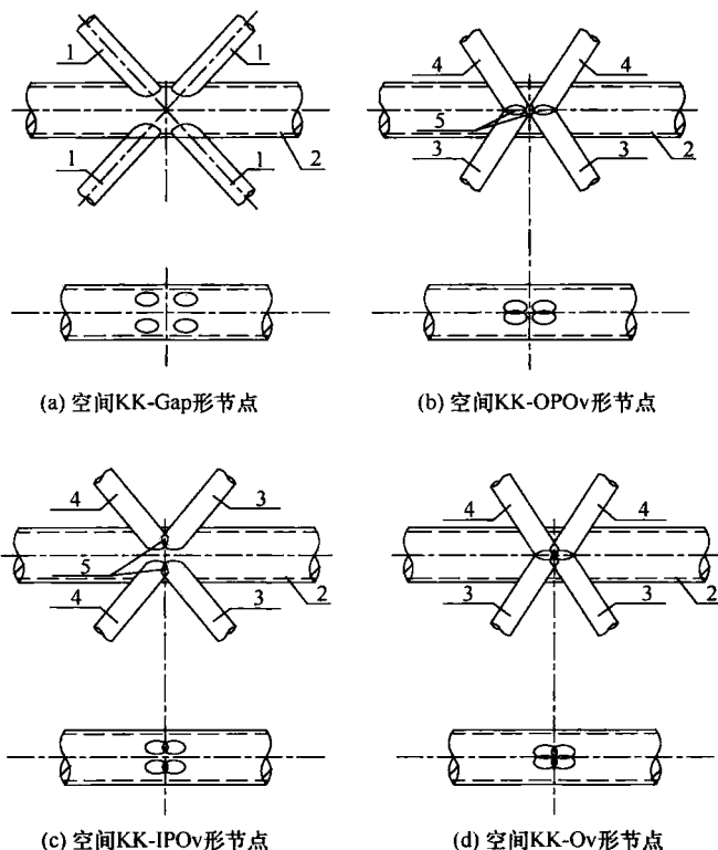
图37 空间KK形节点分类
