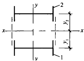
图 8.2.6 格构式构件截面 1—分肢 1；2—分肢 2
