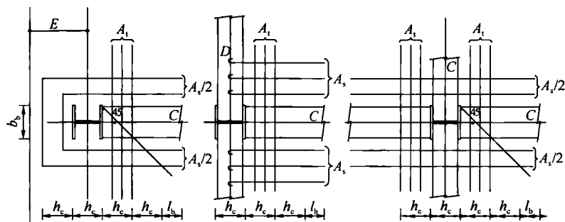
图 50 钢柱周边钢筋锚固示意图
