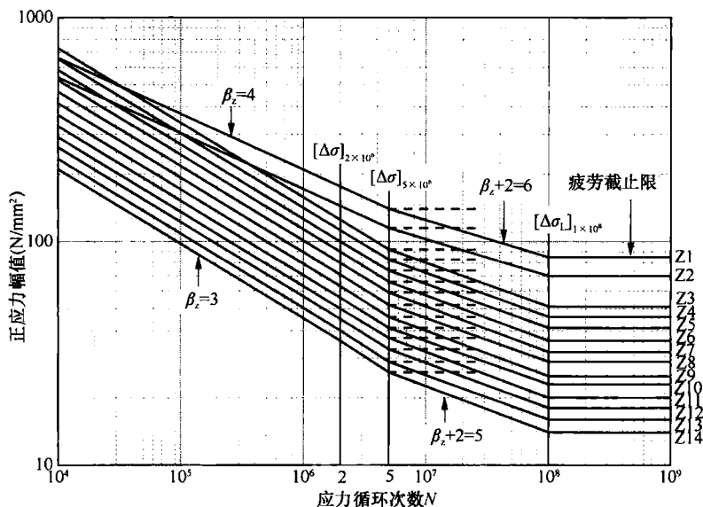
图 46 关于正应力幅的疲劳强度 S-N 曲线
