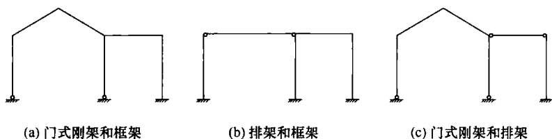
图 51 混合形式
