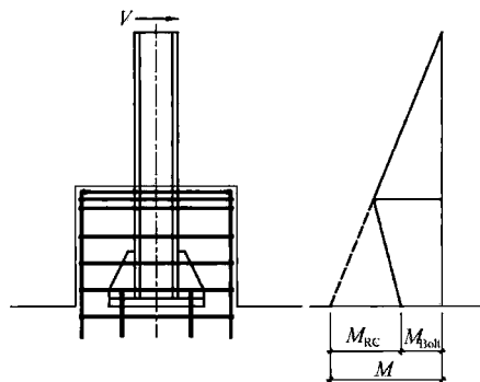
图 24 外包式柱脚地脚螺栓的计算方法
