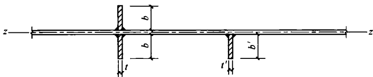
图 4 横向加劲肋的配置方式
