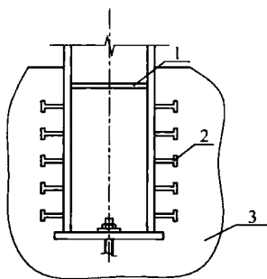
图 25 埋入式柱脚
