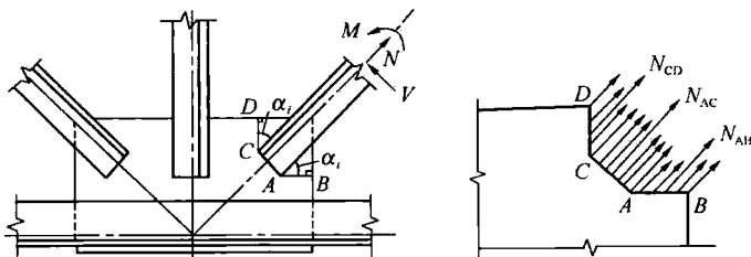
图 17 节点板受拉计算简图
