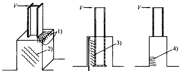
图 22 外包式柱脚的主要破坏模式
