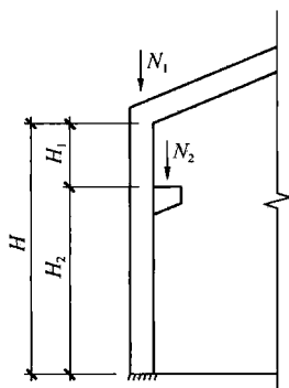
图 8.3.2 单层厂房框架示意
