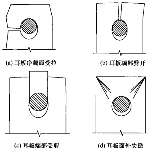
图 16 销轴连接中耳板四种承载力极限状
