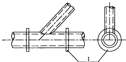
图 35 主管外周设置加劲环的节点
