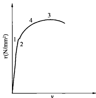
图 15 单个螺栓受剪时的工作曲线
