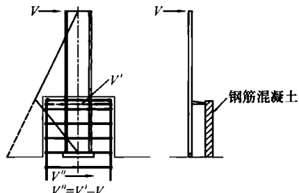
图 21 计算简图
