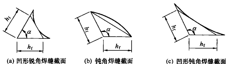
图 11.2.3-1 T 形连接的斜角角焊缝截面
