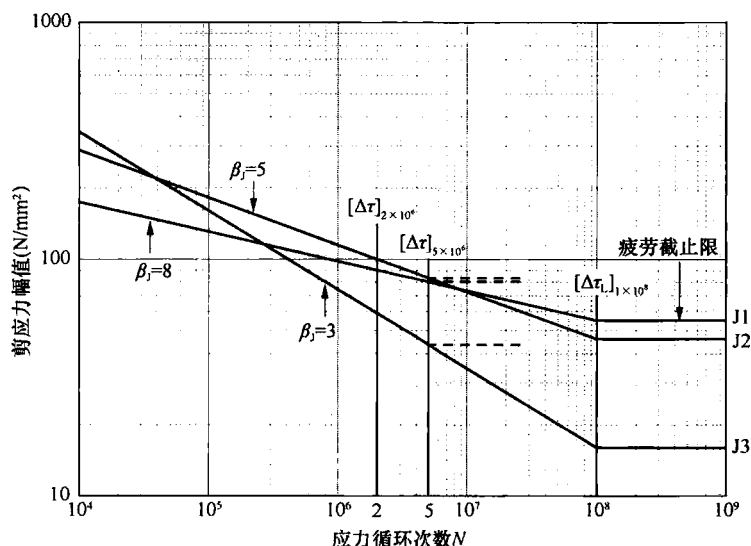
图 47 关于剪应力幅的疲劳强度 S-N 曲线
