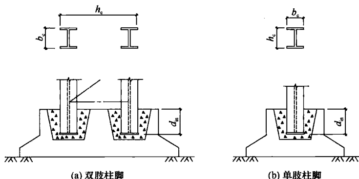
图 26 插入式柱脚
